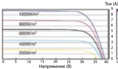
Кривые I-V при различной инсоляции
