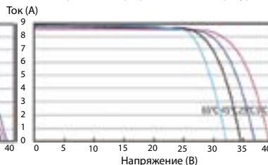
Кривые P-V при различных температурах
